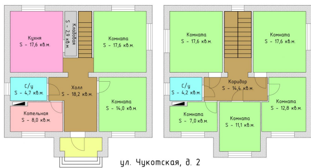
Первый этаж
